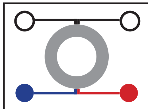
Mantelwellensperre W1JR
