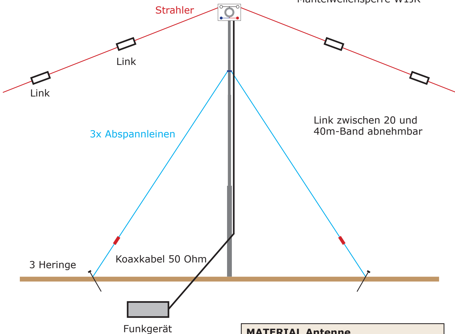
Mantelwellensperre W1JR
